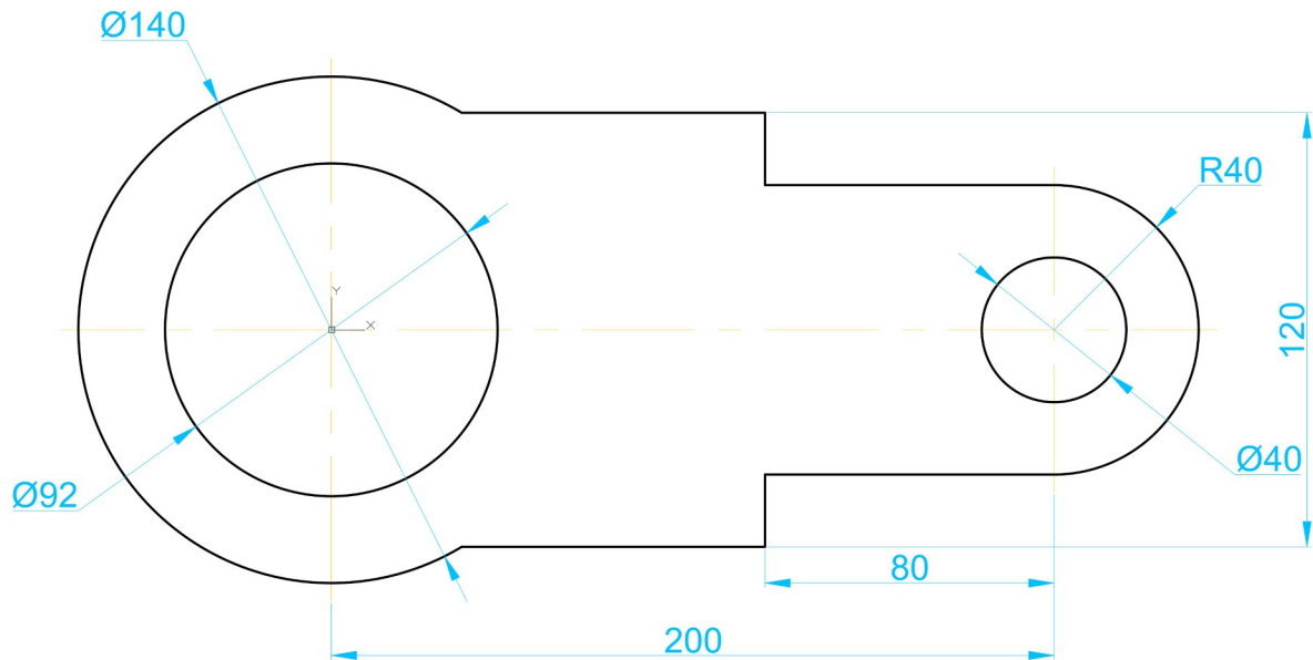
Рисунок 1.1 — Отриманий кресленик
